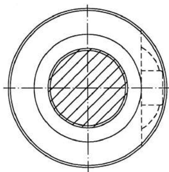
圖 4.1 外循環圓週型
